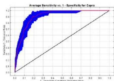
شکل ۱۰: منحنی ROC و مقدار AUC مدل سازی زیستگاه مطلوب کل و بز در پاییز
