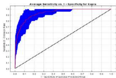
شکل ۹: منحنی ROC و مقدار AUC مدل سازی زیستگاه مطلوب کل و بز در بهار
