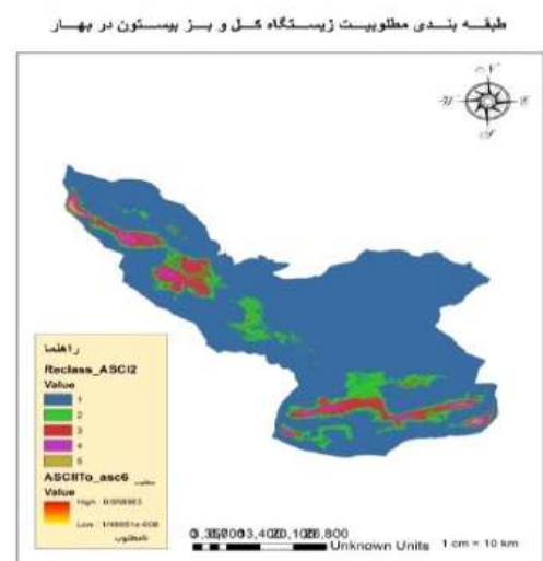
شکل ۱۵: طبقه بندی مطلوبیت زیستگاه کل و بز در منطقه حفاظت شده و پناهگاه حیات وحش بیستون در فصل بهار
