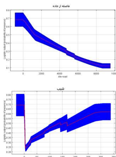
شکل ۵، ۶، ۷ و ۸: منحنی پاسخ به متغیرهای مدل رقومی فاصله از مراکز نظامی - فاصله از مراکز صنعتی - فاصله از جاده - شیب
