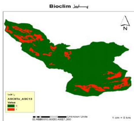
شکل ۲۰: پیش‌بینی مطلوبیت زیستگاه مدل Bioclim در فصل پاییز
