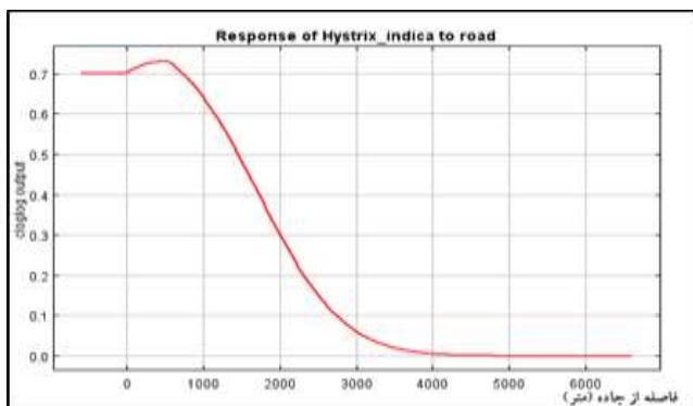
شکل ۵: منحنی پاسخ گونه به فاصله از جاده
