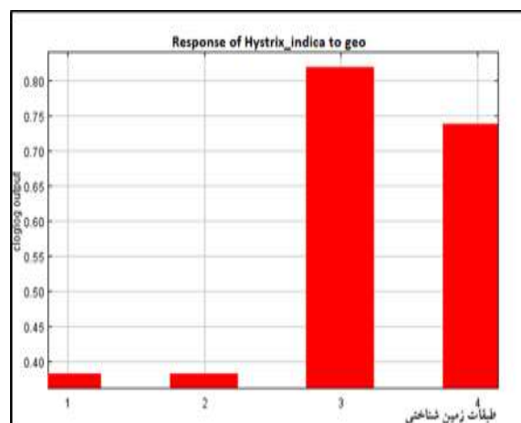
شکل ۱۲: منحنی پاسخ گونه به متغیر زمین شناسی
