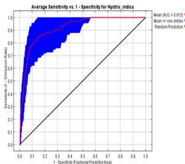
شکل ۱۳: منحنی ROC - شاخص AUC
