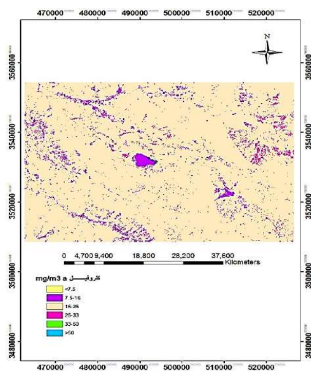
شکل ۱۳: شاخص NDCI در فروردین ماه ۱۳۹۷
