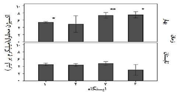
شکل ۸: نمودار اکسیژن محلول
