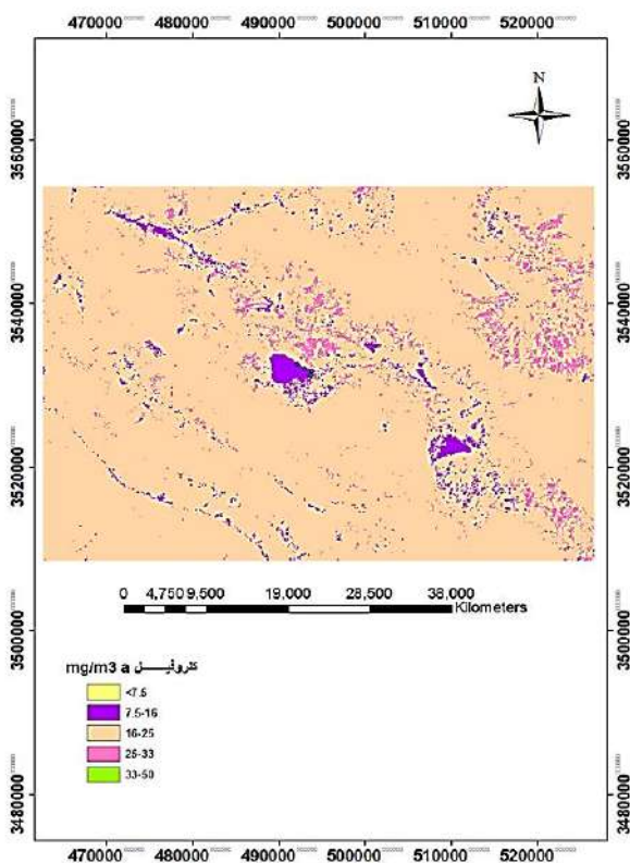
شکل ۱۶: شاخص NDCI در تیرماه ۱۳۹۷
