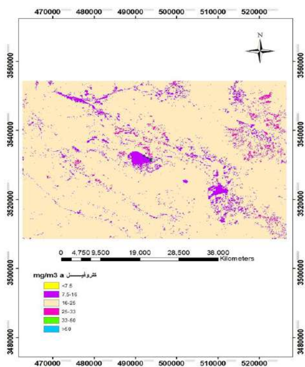
شکل ۱۵: شاخص NDCI در خرداد ماه ۱۳۹۷
