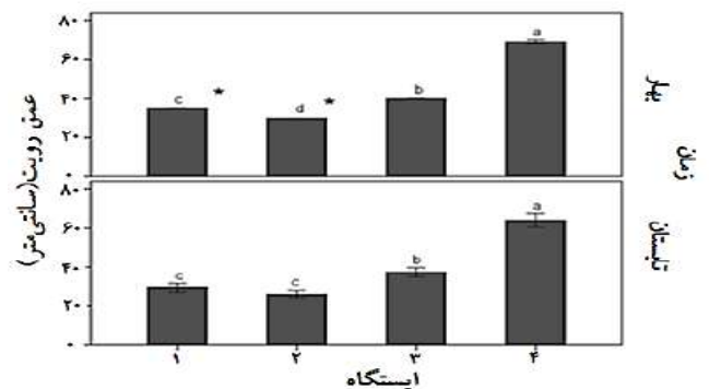
شکل ۱۰: نمودار عمق رویت
