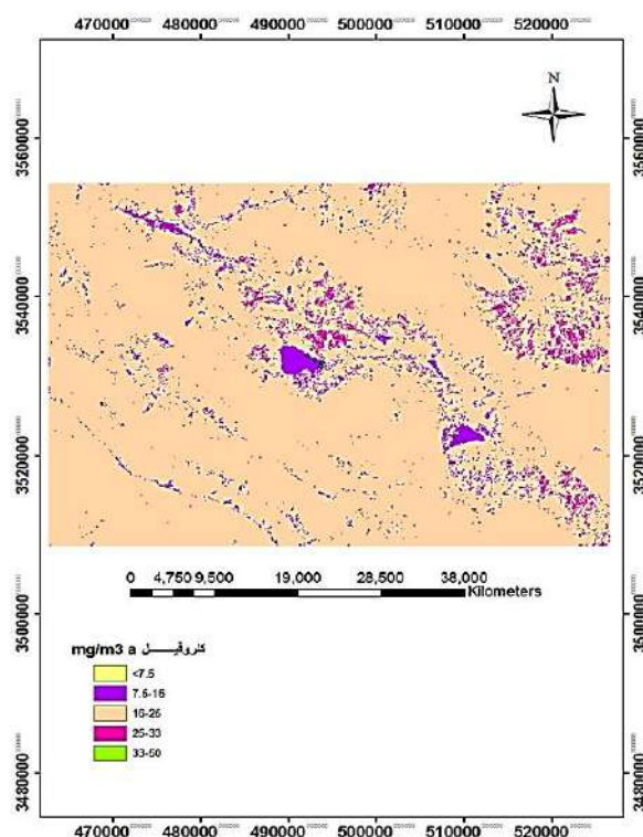
شکل ۱۷: شاخص NDCI در مرداد ماه ۱۳۹۷
