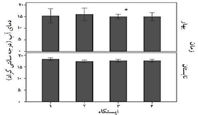
شکل ۴: نمودار درجه حرارت آب
