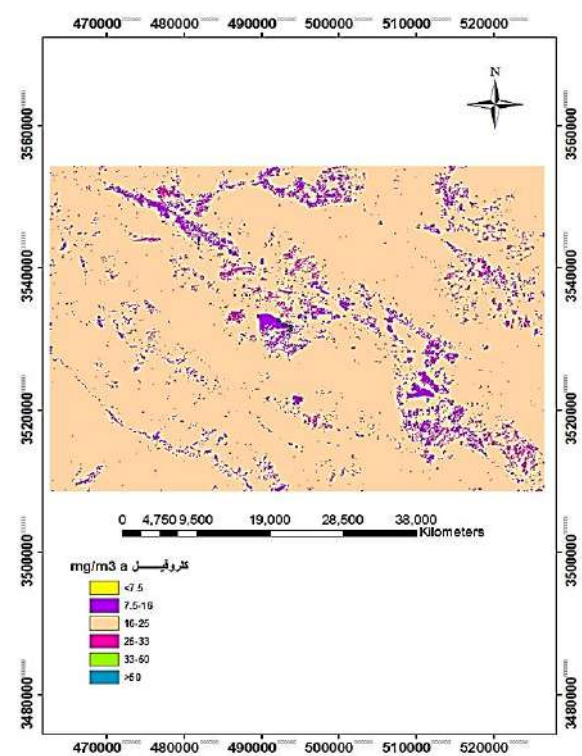
شکل ۱۸: شاخص NDCI در شهریور ماه ۱۳۹۷
