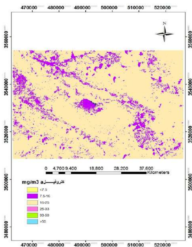
شکل ۱۴: شاخص NDCI در اردیبهشت ماه ۱۳۹۷
